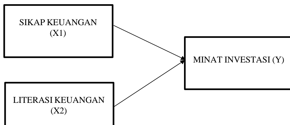
Gambar 1. Kerangka Pemikiran
